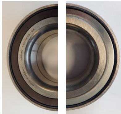
Richtung Innenseite/Außenseite des Fahrzeugs Schwarze Encoder/Metall-Dichtung
