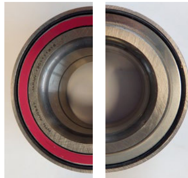
Richtung Innenseite/Außenseite des Fahrzeugs Rosa Metall-Dichtung/Metall-Dichtung
